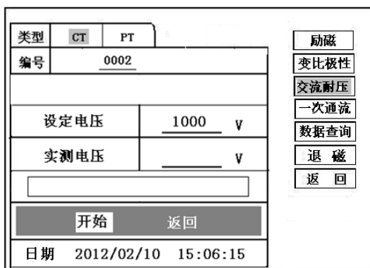
图 16、CT 交流耐压测试界面
