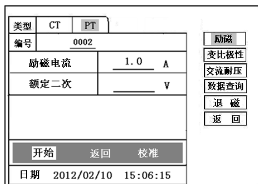
图 18，PT 励磁特性参数设置界面
