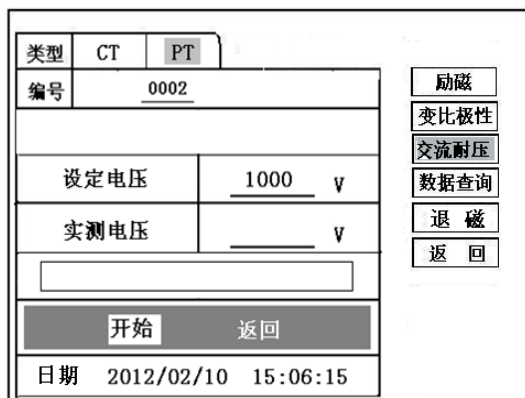
图 23, PT 交流耐压测试界面
